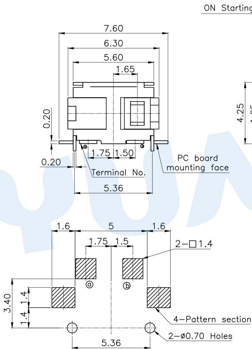
PCB Layout(Pattern side)
