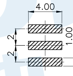
PCB Layout(Pattern Side)
